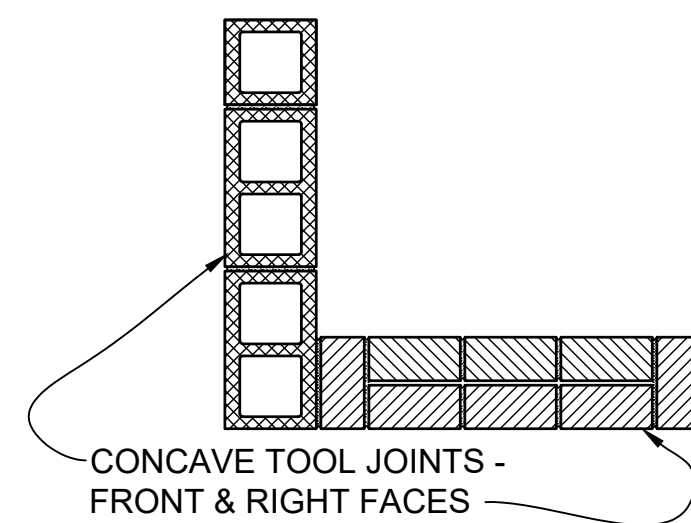
H COURSE 4,6,10,12 3/4"=1'-0"
