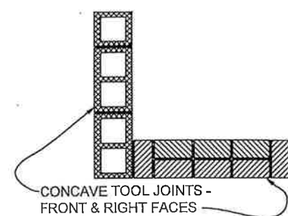
H COURSE 4,6,10,12 3/4"=1'-0"
